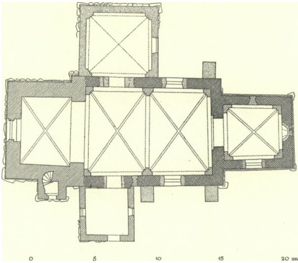
Fig. 2. Gevninge. Plan. 1 : 300. Maalt af C. G. S. 1935.
