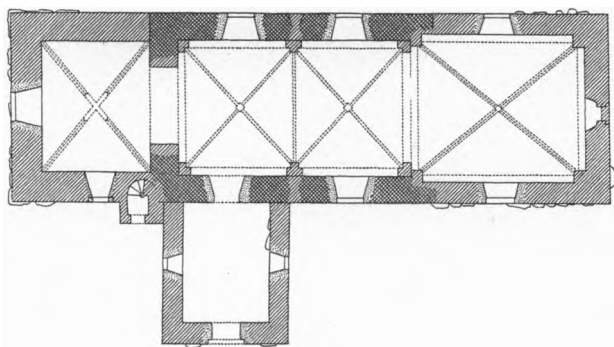
Fig. 2. Jersie. Plan 1:300. Maalt af Knud V. Barfoed 1915 (C. G. S. 1935).
