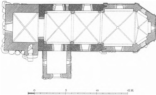
Fig. 2. Solrod. Plan 1:300. Maalt af Knud V. Barfoed 1915 (C. G. S. 1935).
