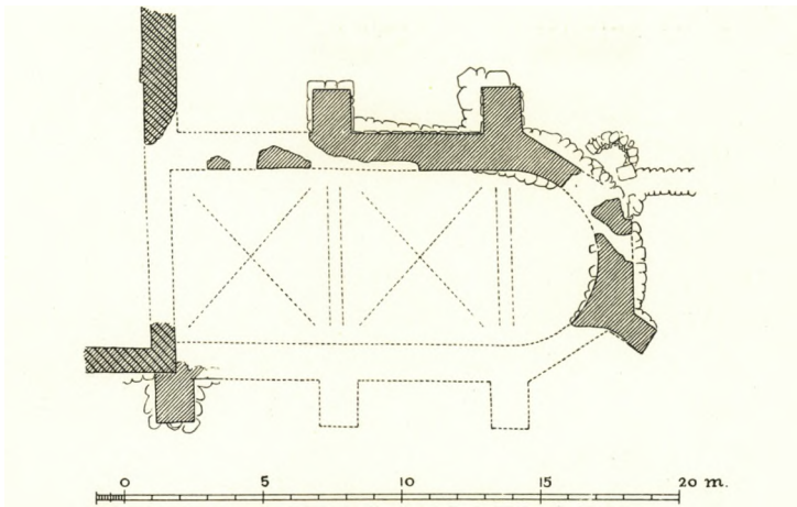
Fig. 1. Roskilde † Bispegaards Kapel. Plan. 1:300. Maalt af El. M. 1941, tegnet af C. G. S. 1944.
