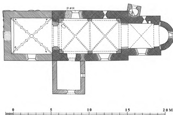
Fig. 3. Plan. 1:300. Målt af MB 1966, tegnet af Marianne Nielsen 1985. Signaturforklaring s. 9. - Ground-plan. Key on p. 9.
