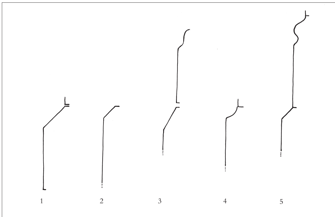
ROMANSKE BYGNINGSPROFILER i Elbo Herred, af granit. 1:10. Målt og tegnet af Anders C. Christensen 2021-22. Fig. 1-5. Bygningssockler. 1. Vejlbj, skibets nordside (frådsten og granit). 2-3. Erritsø, skib og kor. 4. Bredstrup, korets nordside. 5. Taulov, korets østside. – Romanesque building profiles in Elbo District, of granite. Figs. 1-5. Footings.
