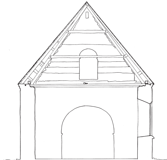
Fig. 4. Tværsnit gennem skib set mod øst. 1:150. Målt og tegnet af Line M. Bonde 2022. – Cross-section through the nave looking east.
