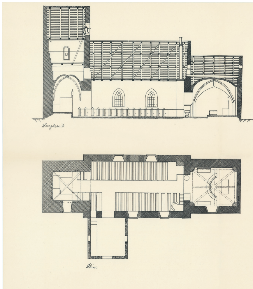
Fig. 13a-b. Opmåling af kirken. 1:300. a. Længdesnit set mod nord. b. Plan. Målt og tegnet af Helge Andreassen 1937. I Kgl. Bygningsinspektors Arkiv. – Scale drawings of the church. a. Longitudinal section looking north. b. Plan.
