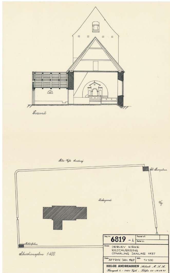
Fig. 13c-d. Opmåling af kirken. c. Tværsnit i skibet set mod vest. 1:300. d. Situationsplan. 1:1200. Målt og tegnet af Helge Andreasen 1937. I Kgl. Bygningsinspektors Arkiv. – Scale drawings of the church. c. Cross-section looking west. d. Plan of churchyard.
