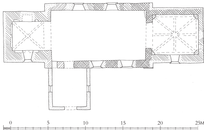
Fig. 3. Grundplan. 1:300. Målt af Helge Andreassen 1937, suppleret og tegnet af Line M. Bonde 2022. Signaturforklaring s. 9. – Plan. Key on p. 17.
