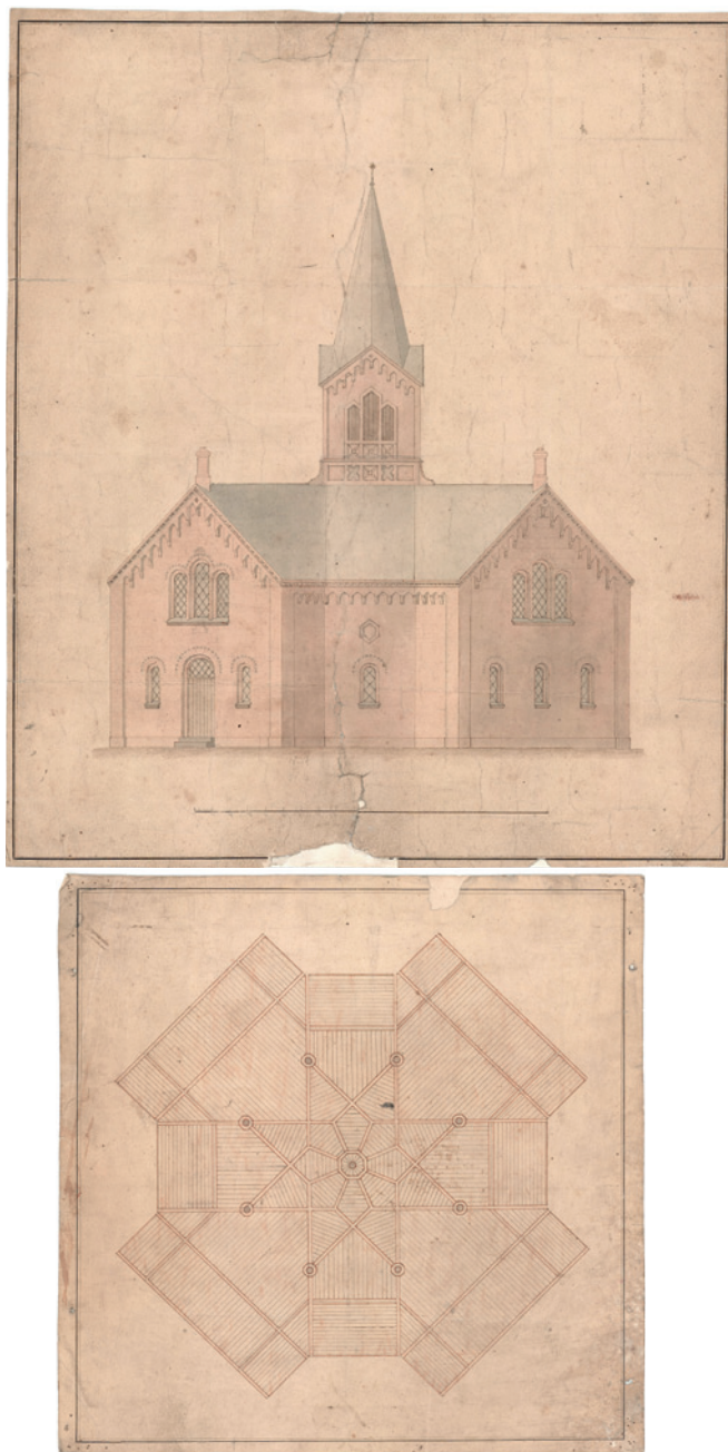
Fig. 8a-d. Snit, grundplan, opstalt og loftsplan. 1:300. Bygningstegninger ved Andreas Bentsen til valgmenighedskirken i Vallekilde 1880, genbrugt i Balle. I Danmarks Kunstbibliotek. – Cross-section, ground plan, elevation and ceiling plan.
