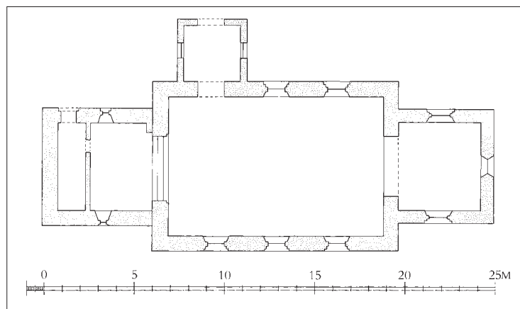
Fig. 5. Plan. 1:300. Målt af P. Bruhn og Søn, 1980. Suppleret af Niels Jørgen Poulsen og tegnet af Freerk Oldenburger 2017. Signaturforklaring s. 9. – Ground plan. Key on p. 17.
