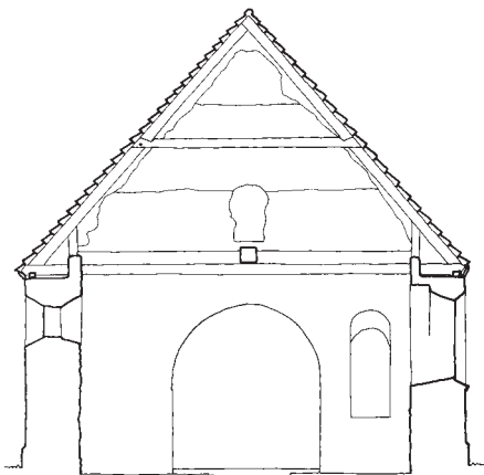
Fig. 5. Tværsnit gennem skib set mod øst. 1:150. Målt af Anders C. Christensen og Jakob Kieffer-Olsen, tegnet af Anders C. Christensen 2017. – Cross-section through nave looking east.
