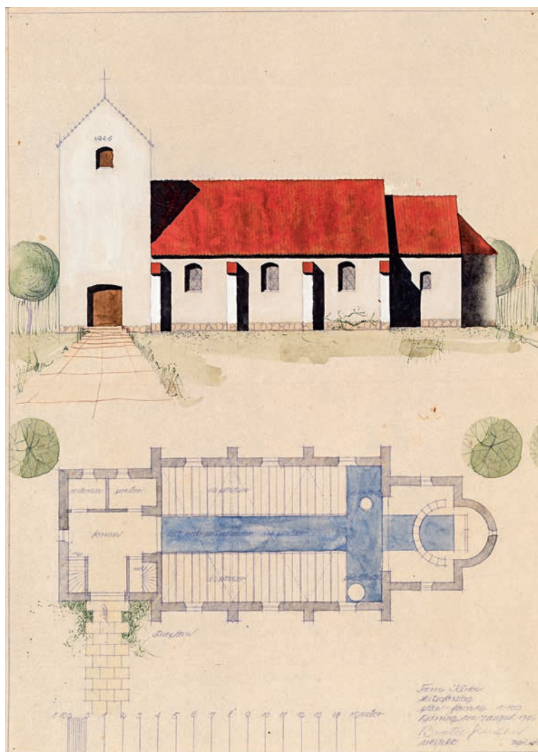
Fig. 7a-c. Ikke anvendt projekt til kirke. 1:300. Tegnet af Bertel Jensen, 1946. Give-Egnens Museum og arkiv. a. Sydfacade og plan. b. Vest- og østfacade samt tværsnit af skib set mod vest og kor set mod øst. c. Længdesnit set mod nord. – Unused proposal for a church, 1946. a. South facade and ground plan. b. West and east facade; cross-sections through nave and chancel. c. Longitudinal section.
