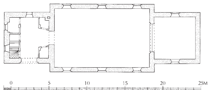
Fig. 4. Grundplan. 1:300. Bertel Jensen 1955, suppleret af Jakob Kieffer-Olsen og tegnet af Freerk Oldenburger 2016. – Ground plan.
