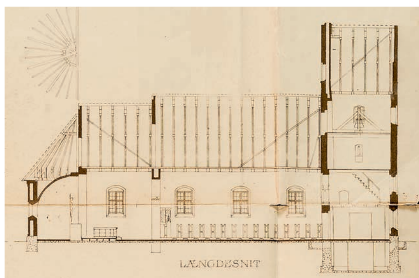
Fig. 6a-f. Ikke anvendt projekt til kirke. 1:300. Tegnet af Axel Hansen, 1928. Give-Egnens Museum og arkiv. a. Længdesnit set mod syd. b. Nordfacade. c. Tværsnit af tårnet set mod øst. d. Sydfacade. e. Tværsnit af skibet set mod vest. f. Plan. – Unused proposal for a church, 1928. a. Longitudinal section. b. North facade. c. Cross-section of tower. d. South facade. e. Cross-section of nave. f. Ground plan.
