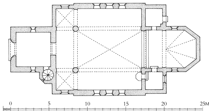
Fig. 3. Grundplan. 1:300. Tegnet af Merete Rude 2011 efter Johs. Magdahl Nielsen 1911. – Ground plan.
