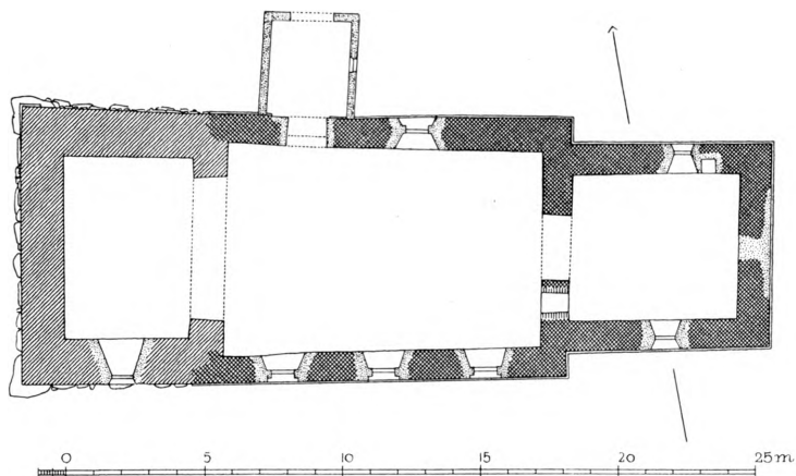
Fig. 2. Solbjærg. Plan. 1:300. Maalt af C. G. Schultz 1940.
