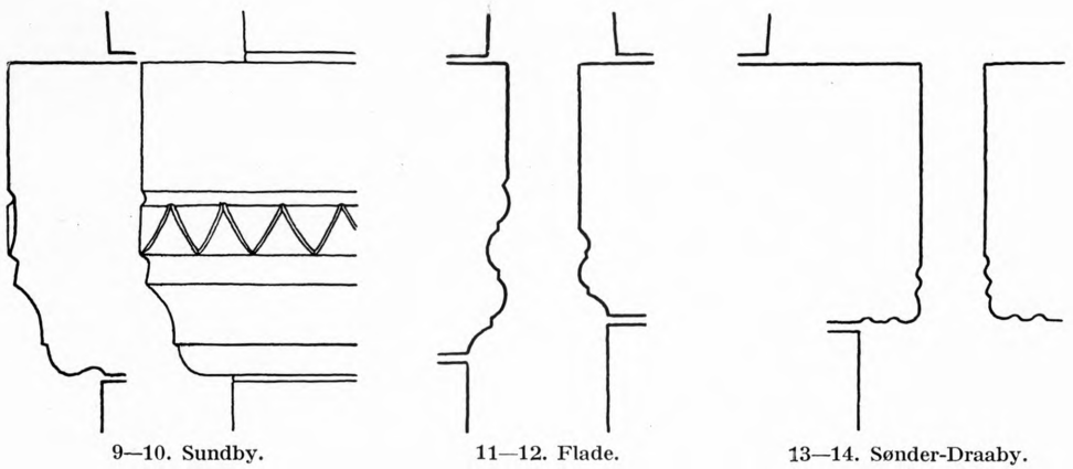
Fig. 1—14. Romanske Bygningsprofiler i Morsø Nørre-Herred. 1:10. Maalt af C. G. Schultz. Korbuer.
