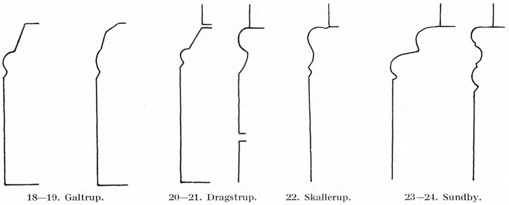
Fig. 15—24. Romanske Bygningsprofiler i Morsø Nørre-Herred. 1:10. Maalt af C. G. Schultz. Fig. 15—17 Korbuer. Fig. 18, 19 og 22 udvendige Sökkeler. Fig. 20—21 og 23—24 Korbuesökkeler.
