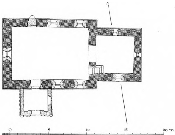
Fig. 2. Tæbring. Plan. 1 : 300. Maalt af C. G. Schultz 1940.
