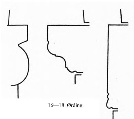
Fig. 1—18. Romanske Bygningsprofiler i Morsø Sønder-Herred. 1:10. Maalt af C. G. Schultz. 1, 3—10, 15 og 17 Korbuekragsten. 2 Dørkarm. 11 og 18 Apsisbuekragsten. 12 Konsolsten. 13 og 16 Taarnbuekragsten. 14 Portalkragsten.
