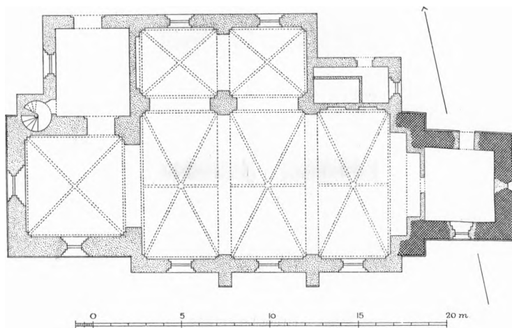
Fig. 3. Jegindø. Plan, efter Ombygningen 1919. 1:300. Maalt af C. G. Schultz 1938.
