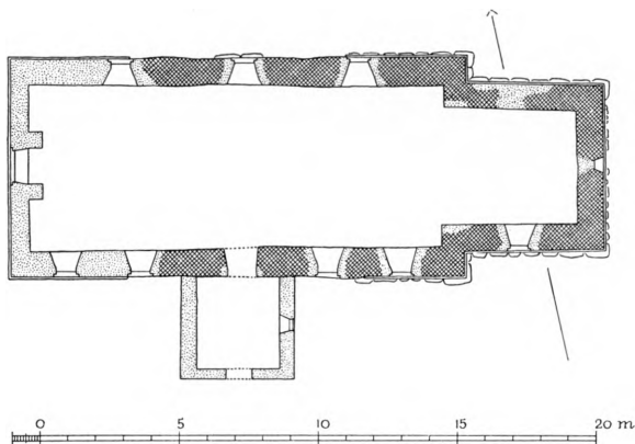
Fig. 2. Jegindø. Plan, før Ombygningen 1919. 1:300. Maalt af Hother Paludan 1918 (C. G. Schultz).
