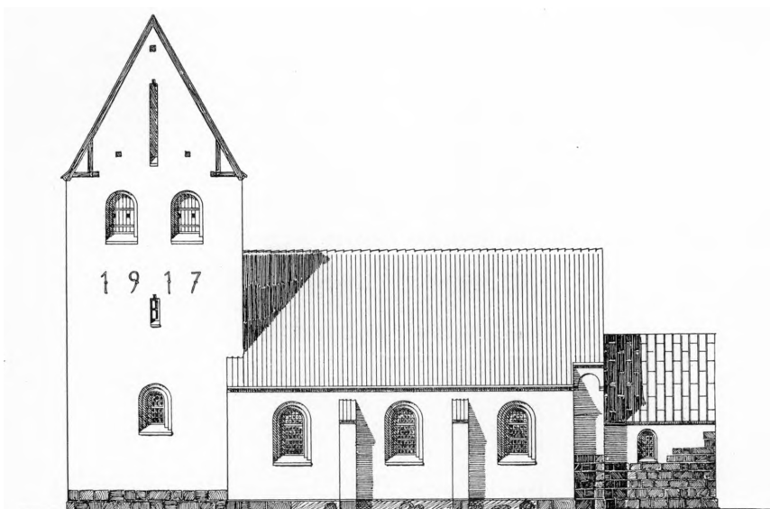
Fig. 1. Jegindø. Opstalt. 1:300. Set fra Syd. Udkast af Hother Paludan 1916.
