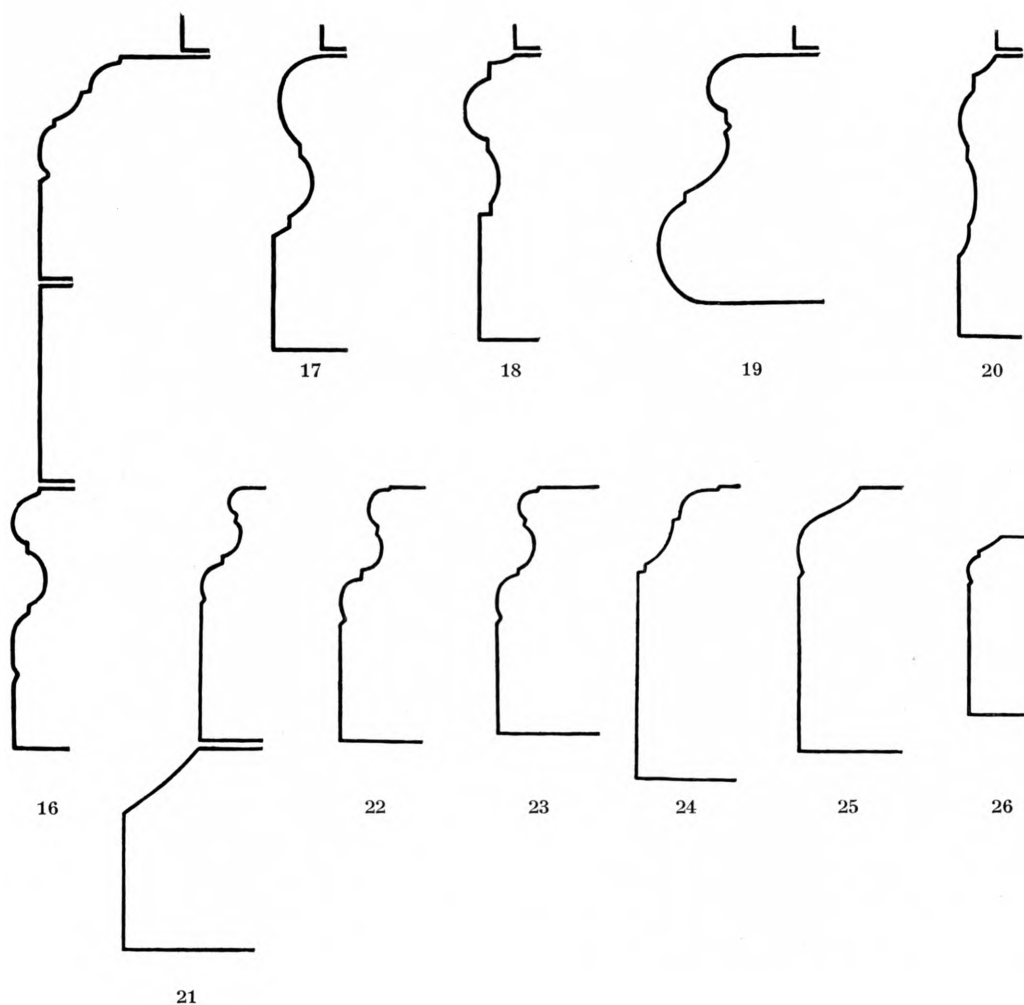
Fig. 1—26. Romanske Bygningsprofiler i Vestervig, Revs Herred. 1 : 10. (C. G. Schultz).
