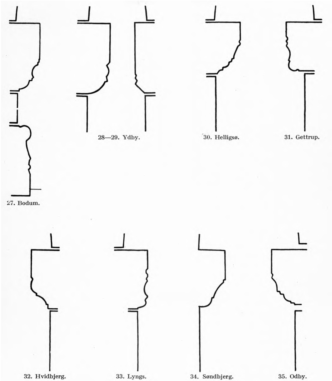
Fig. 27—35. Romanske Bygningsprofiler (Korbuer) i Revs Herred. 1:10. (Se ogsaa under Hurup). Maalt af C. G. Schultz.
