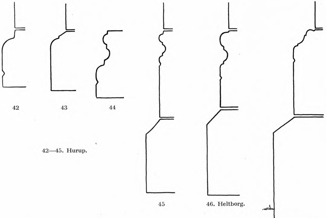
Fig. 36—47. Romanske Bygningsprofiler (Sokler) i Revs Herred. 1:10. Maalt af C. G. Schultz.
