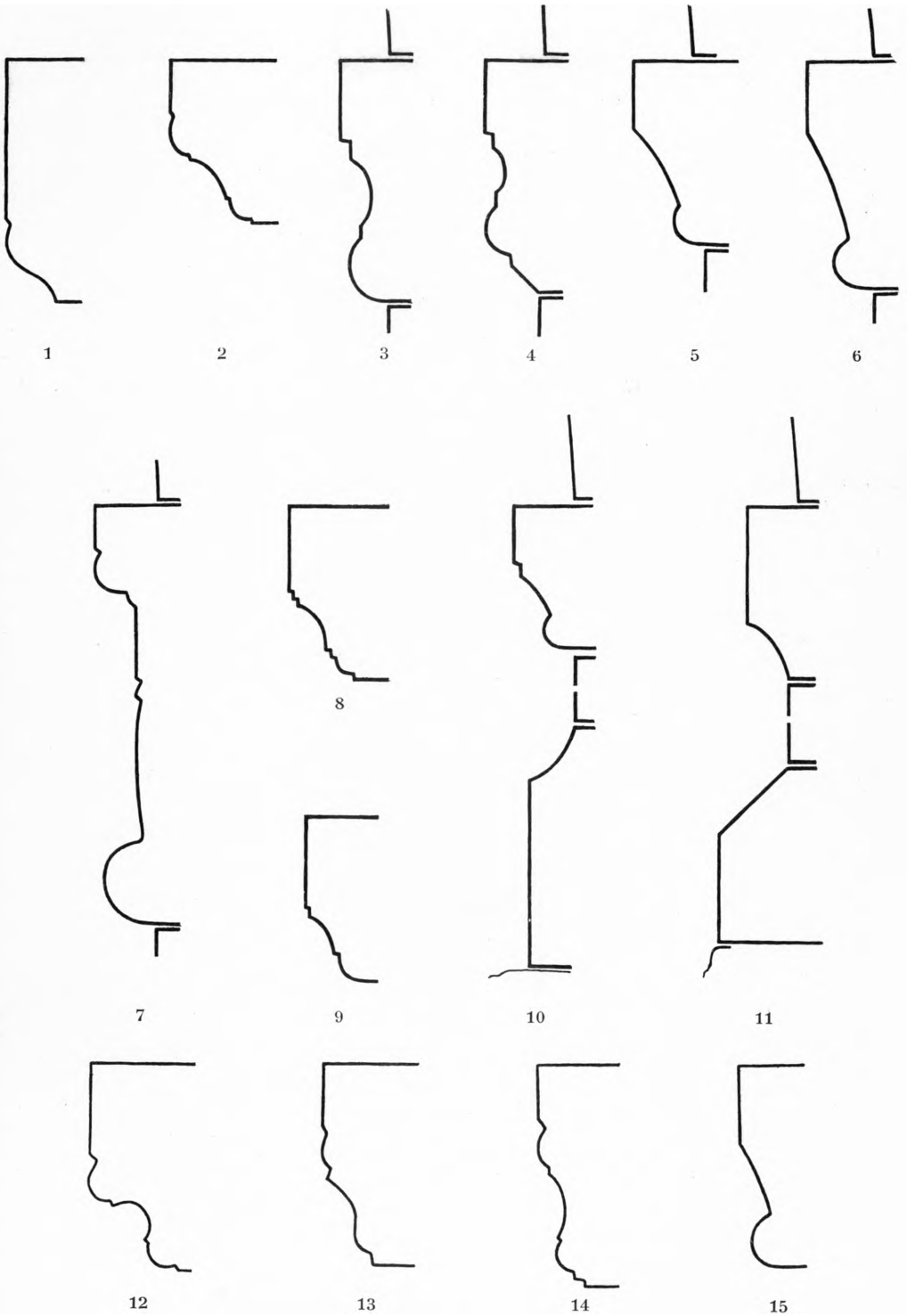
Fig. 1—15. Romanske Bygningsprofiler i Vestervig, Revs Herred. 1:10. (C. G. Schultz), (sml. S. 606).
