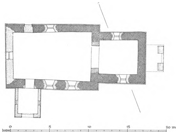
Fig. 2. Grurup. Plan. 1:300. Maalt af C. G. Schultz 1937.
