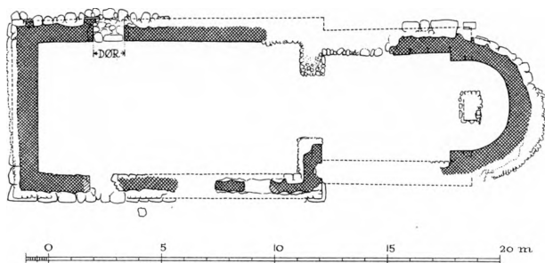
Fig. 2. †Torup. Plan. 1:300. Maalt af C. G. Schultz 1940.
