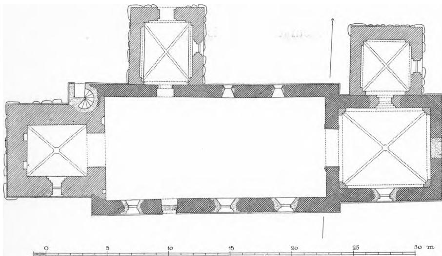
Fig. 2. Sennels. Plan. 1 : 300. Maalt af C. G. Schultz 1936; med Tilføjelser efter J. Foged 1937.
