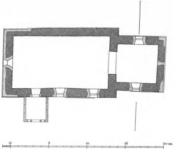
Fig. 2. Kaastrup. Plan 1 : 300. Maalt af C. G. Schultz 1936.
