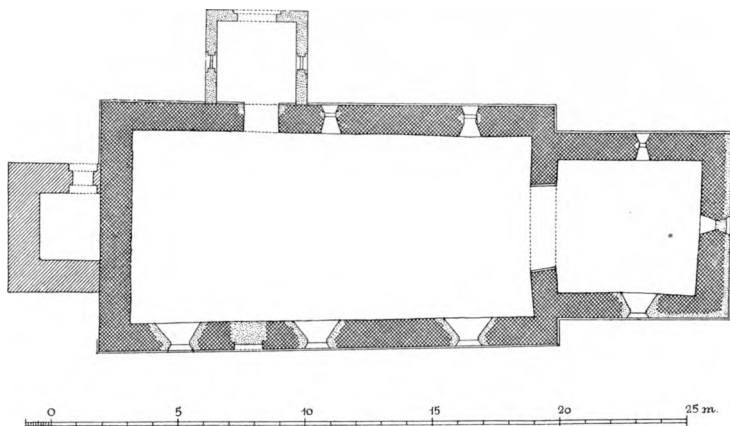
Fig. 3. Tved. Plan. 1 : 300. Maalt af C. G. Schultz 1936.
