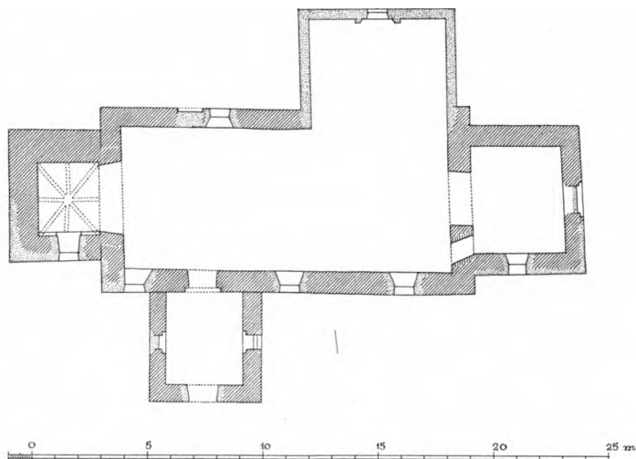
Fig. 2. Lild. Plan. 1:300. Maalt af C. G. Schultz 1936.
