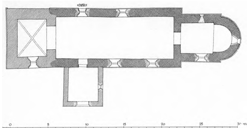
Fig. 2. Gøttrup. Plan. 1:300. Maalt af C. G. Schultz 1936.
