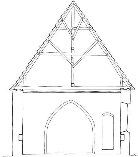
Fig. 8. Tværsnit. 1:150. Målt af Knud Lehn Petersen 1923, suppleret og tegnet af Pia K. Lindholt 2023. – Cross-section.
