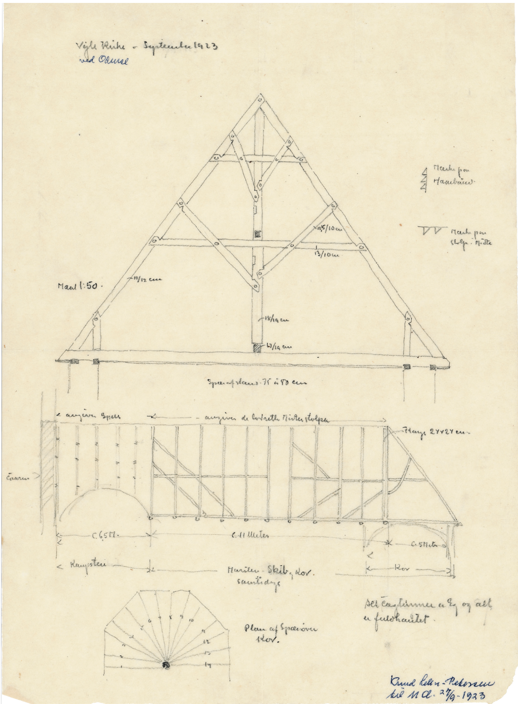
Fig. 25a-c. Opmåling af langhusets tagværk. a. Tværsnit. 1:150. b. Længdesnit. c. Plan. Målt og tegnet af Knud Lehn Petersen 1923. I NM. — Scale drawing of the roofing of the nave church. a. Cross-section. b. Longitudinal section. c. Plan.
