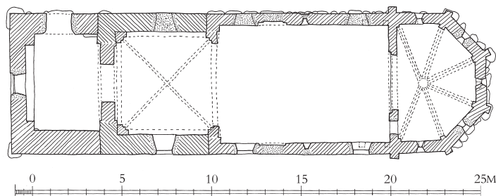
Fig. 7. Grundplan. 1:300. Målt af Ebbe Lehn Petersen 1962, suppleret og tegnet af Pia K. Lindholt 2023. Signaturforklaring s. 9. – Ground plan. Key on p. 17.
