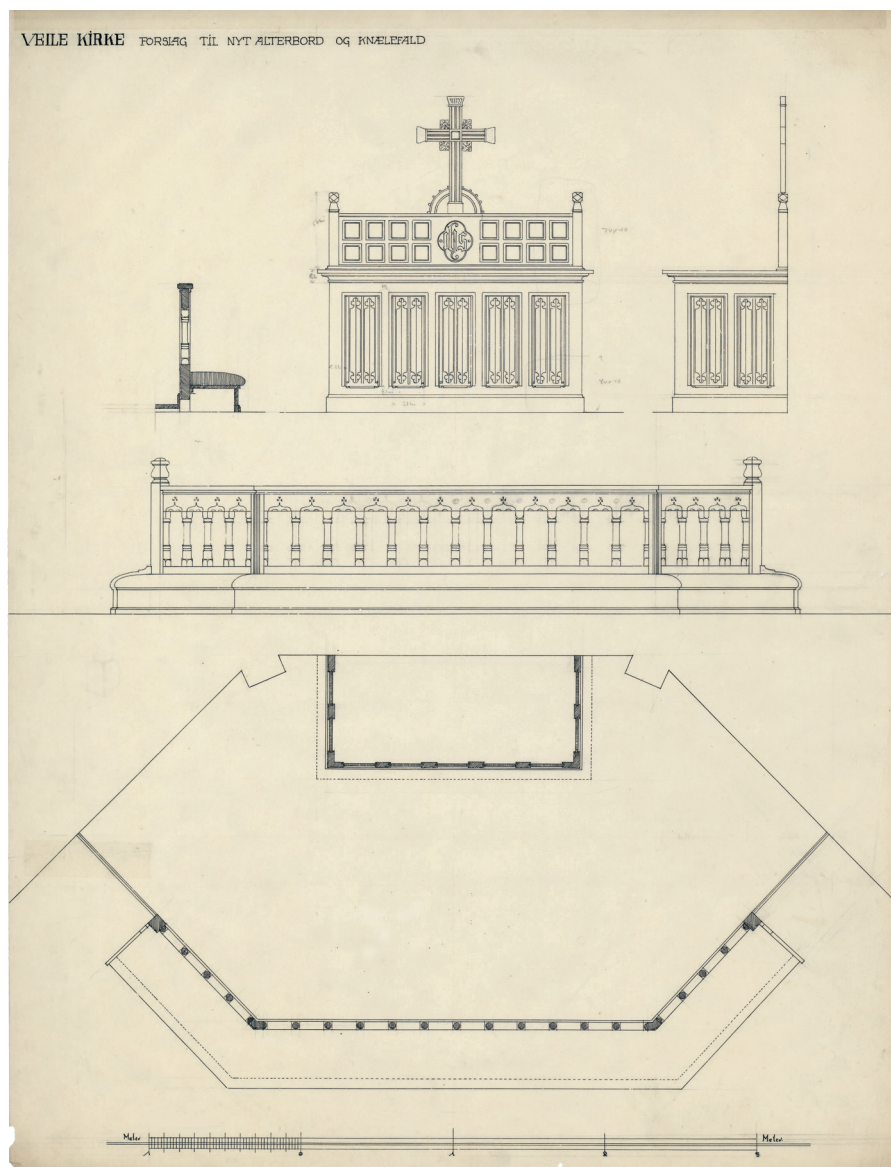
Fig. 40. Forslag til nyindretning af koret 1924 med alterbord, (†)alterudsmykning nr. 3 og †alterskranke (s. 3943, 3947 og 3951). 1:50. Tegnet af Knud Lehn Petersen. I NM. – Proposal for refurnishing of the chancel, 1924, with Communion table, (†)altar decoration no. 3 and †altar rail.
