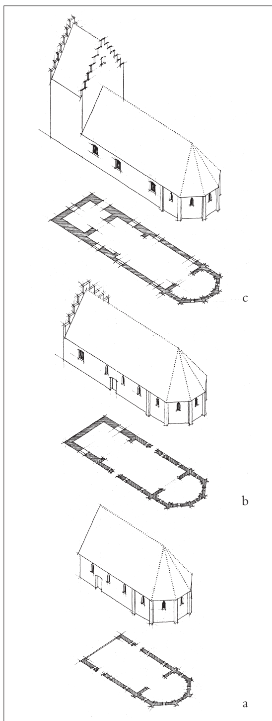
Fig. 22a-c. Rekonstruktion af kirkens byggefaser. 1:600. a. Ungotisk. b. O. 1492. c. Senmiddelalderlig. Tegnet af Ebbe Lehn Petersen o. 1962. I NM. – Reconstruction of the church's construction phases. a. Early Gothic. b. C. 1492. c. Late medieval.
