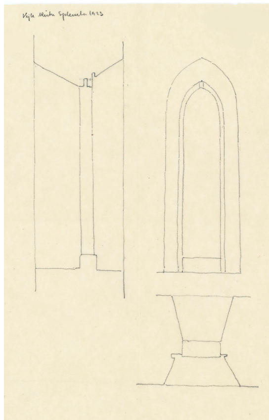
Fig. 65. Opmåling af ungotisk vindue i koret (s. 3921). Målt og tegnet af Knud Lehn Petersen 1923. I NM. – Scale drawing of Early Gothic window in the chancel.
