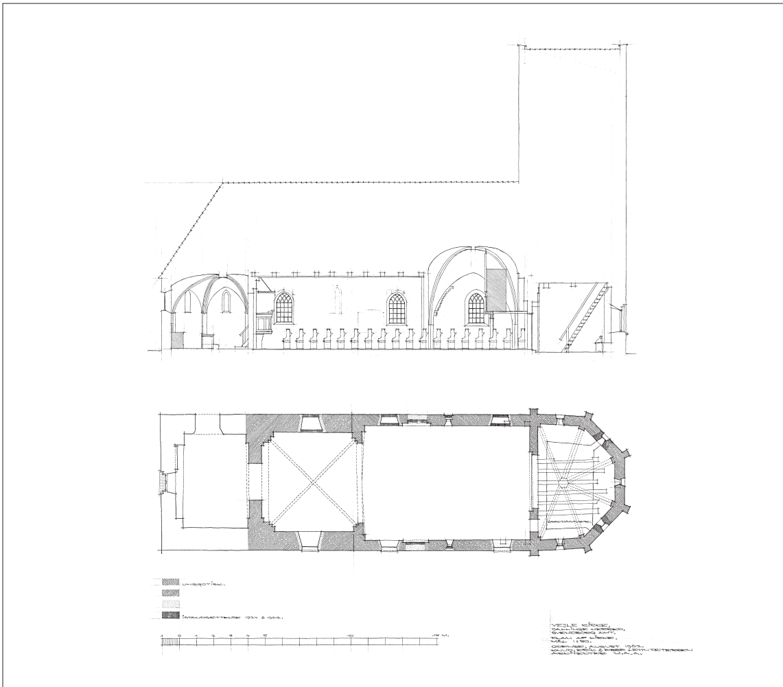
Fig. 23-24. Opmålinger. 1:300. 23. Længdesnit. Målt og tegnet af Erik og Ebbe Lehn Petersen 1959. I NM. 24. Grundplan. Målt og tegnet af Knud, Erik og Ebbe Lehn Petersen 1962. I NM. – 23. Longitudinal section, 1959. 24. Ground plan, 1962.
