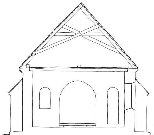
Fig. 10. Tværsnit. 1:150. Målt af Lehn Petersens Tegnestue 1996, suppleret og tegnet af Pia K. Lindholt 2023. – Cross-section.
