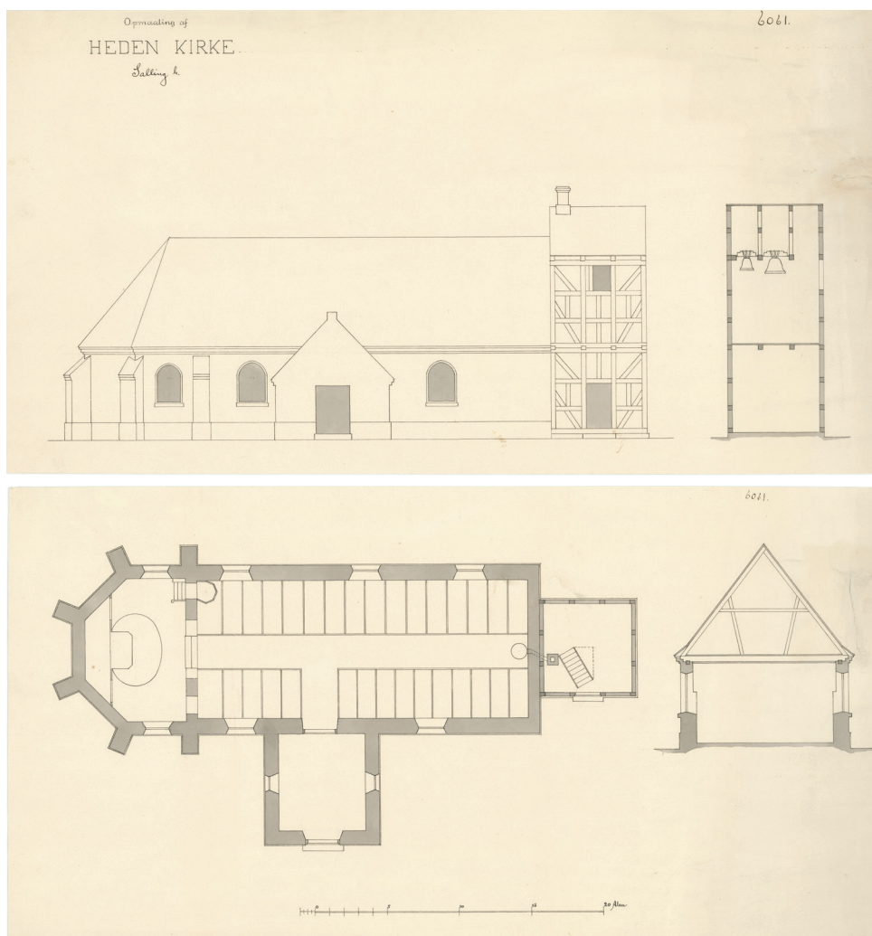
Fig. 15a-d. Opmåling af kirken inden ombygningen 1886-87. 1:300. a. Opstalt set fra nord. b. Tværsnit gennem tårnet. c. Plan. d. Tværsnit gennem skibet. Formentlig tegnet af Hans Fussing o. 1886. I NM. – Scale drawing of the church before rebuilding of 1886-87. a. Elevation seen from the north. b. Cross-section through tower. c. Plan. d. Cross-section through nave.
