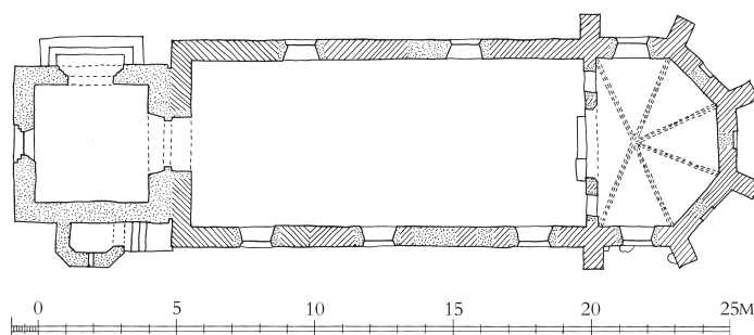
Fig. 9. Grundplan. 1:300. Målt af Lehn Petersens Tegnestue 1996, suppleret og tegnet af Pia K. Lindholt 2023. Signaturforklaring s. 9. – Ground plan. Key on p. 17.
