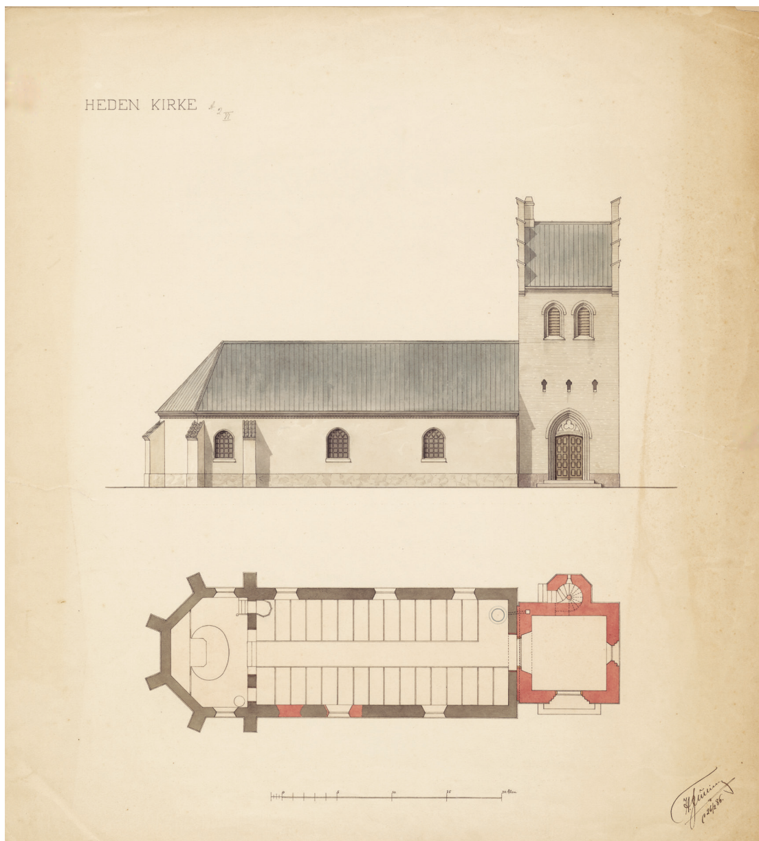
Fig. 16a-b. Tegninger til kirkens ombygning, 1:300. a. Opstalt set fra nord. b. Plan. Tegnet af Hans Fussing 1885-86. I Danmarks Kunstbibliotek. —Drawings for the rebuilding of the church. a. Elevation seen from the north. b. Plan.
