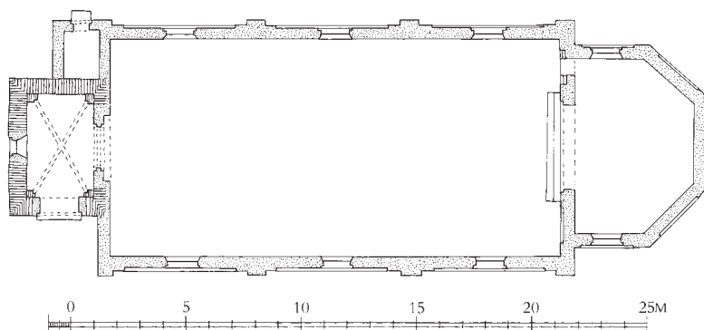
Fig. 7. Grundplan. 1:300. Målt og tegnet af Pia K. Lindholt 2020. Signaturforklaring s. 9. – Ground plan. Key on p. 17.
