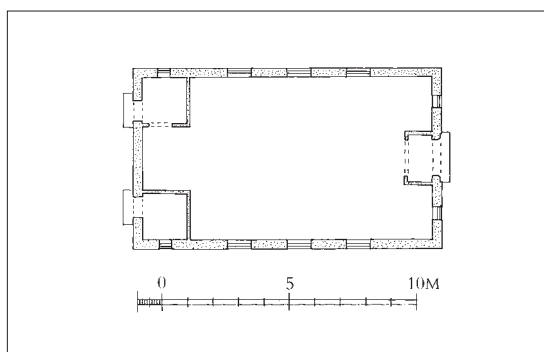
Fig. 3. Grundplan. 1:300. Målt af Lars Mindedal 1988, suppleret og tegnet af Pia K. Lindholt 2020. Signaturforklaring s. 9. – Ground plan. Key on p. 17.
