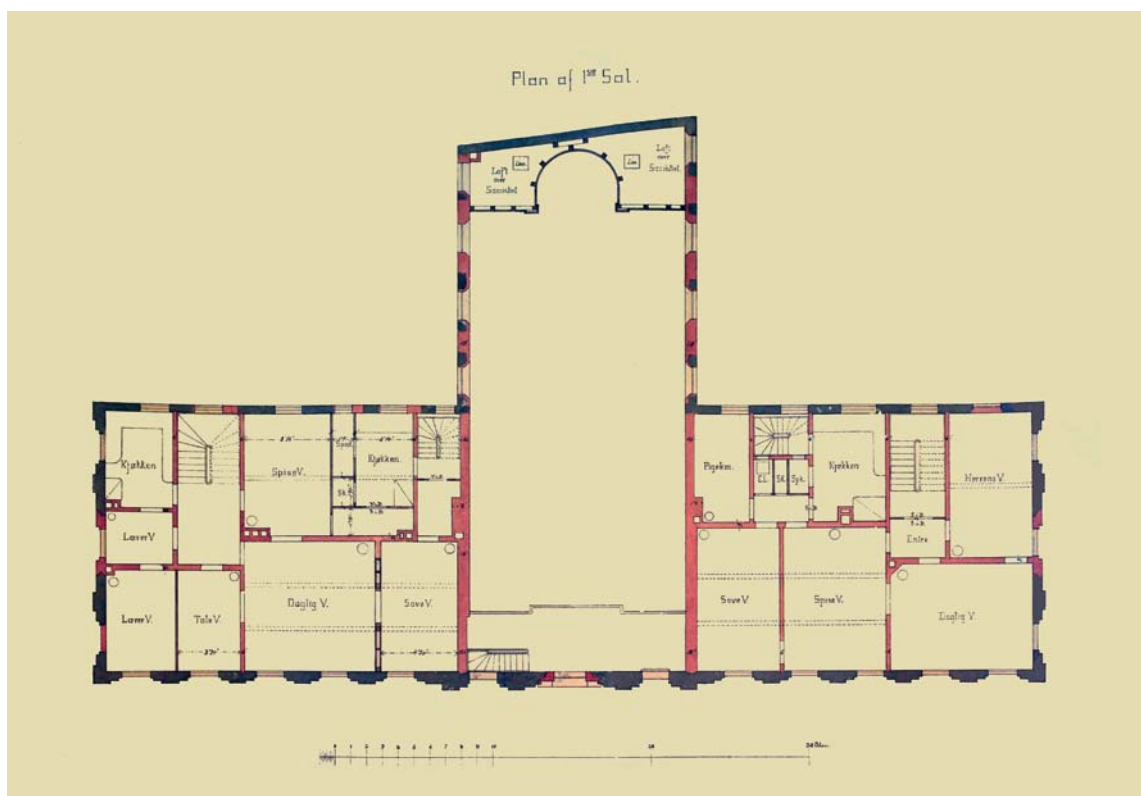
Fig. 1. Forslag til indretning af kirke i den tidligere cikoriefabrik, plan af 1. sal. 1:300. Kirken er beliggende i midtfløjen med højaltret mod nord. Tegning af Ludvig Knudsen 1887. I Katolsk Arkiv, København. – Proposal for the furnishing of the church in the former chicory factory. Plan of first floor. The church is in the middle wing with the high altar to the north.
