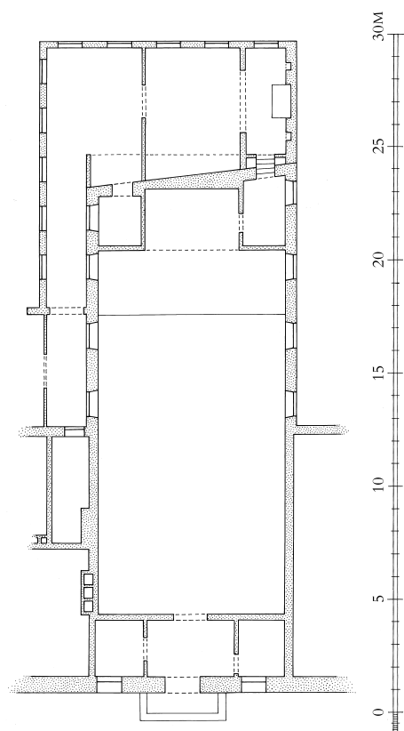
Fig. 2. Grundplan. 1:300. Tegnet af Merete Rude 2012 efter I. Arthur-Nielsen 1969, suppleret af Niels Jørgen Poulsen. – Ground plan.
