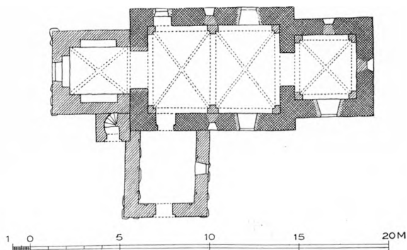
Fig. 2. Gudum. Plan. 1 : 300. Maalt af K. V. Barfoed 1915 (Aage Roussell 1932).
