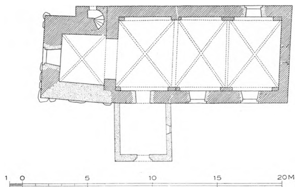
Fig. 2. Farendlose. Plan. 1:300. Maalt af K. V. Barfoed 1913 (C. G. Schultz 1937).
