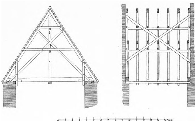
Fig. 3. Nordrup. Taarnets Tagværk 1 : 150. Maalt af K. V. Barfoed 1913.
