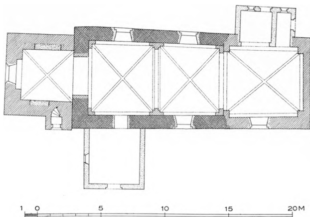
Fig. 2. Nordrup. Plan. 1 : 300. Maalt af K. V. Barfoed 1913 (C. G. Schultz 1931).
