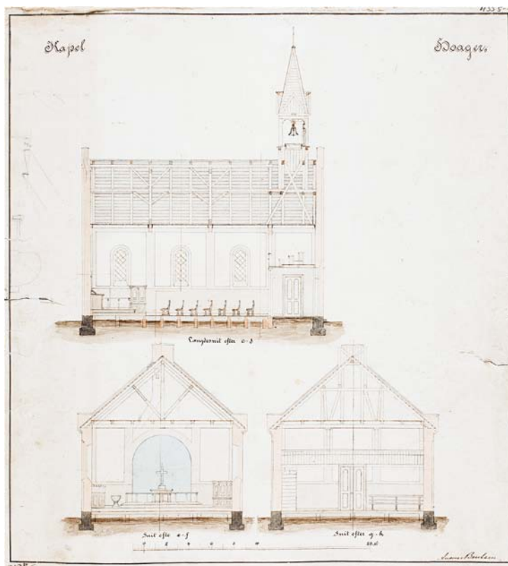
Fig. 2b. Snit. 1:300. Målt og tegnet af Andreas Bentsen 1899. Holstebro Lokalhistoriske Arkiv. – Schnitt .
