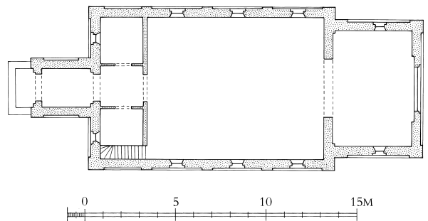
Fig. 3. Plan 1:300. Målt af H. Møller Nielsen 1976, tegnet af Merete Rude 2013. – Grundriss.
