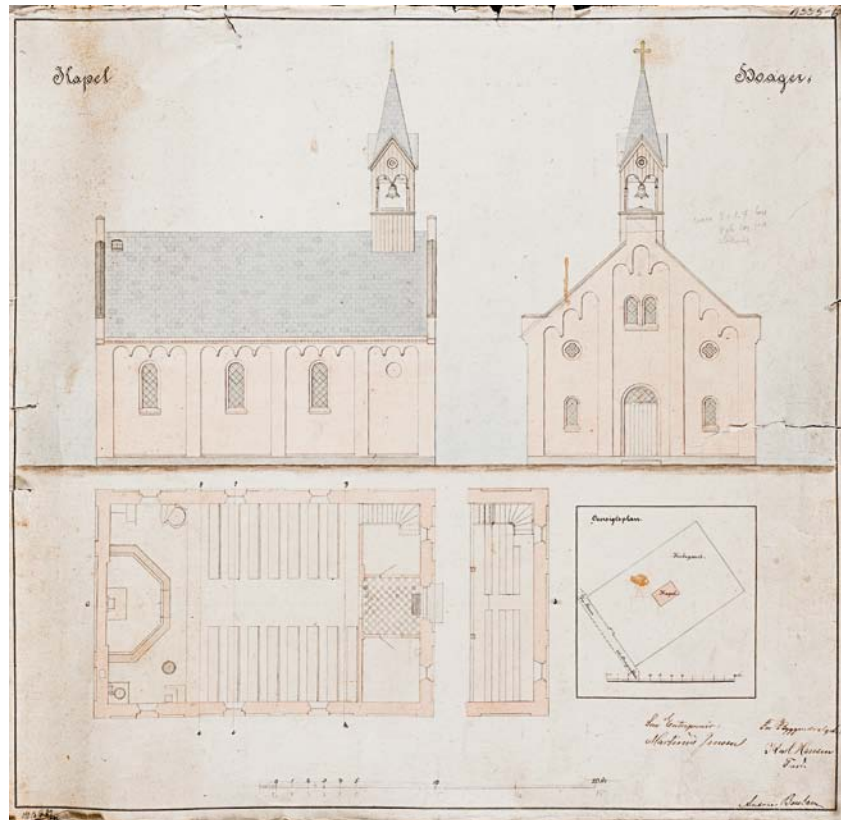
Fig. 2a. Plan og og facader. 1:300. Målt og tegnet af Andreas Bentsen 1899. Holstebro Lokalhistoriske Arkiv. – Grundriss und Fassaden.
