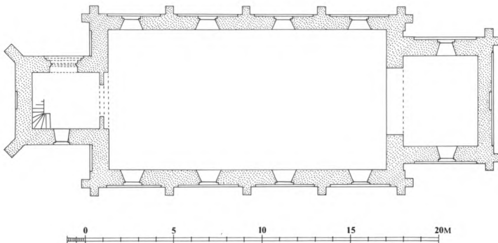
Fig. 2. Grundplan 1:300. Tegnet af Marianne Nielsen 1991 efter skitse-mæssig opmåling af Jens Vilhelmsen 1989, suppleret af Niels Jørgen Poulsen 1991. – Grundriss .
