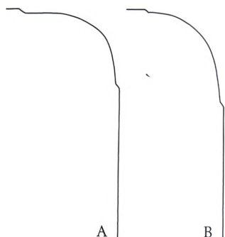
Fig. 2. Profiler af romanske sokkelkvadre, sandsynligvis fra den nedbrudte kirke i Fitting (s. 2302 og 2332). A. Genanvendt i soklen i Vorbasse kirkes søndre korsarm. B. Brugt som gravsten, 1962, på Vorbasse kirkegård, efter at den tidligere havde ligget som trappesten på en gård i Fitting. 1:5. Målt og tegnet af NJP og MN, 1985 og 1990. – Profile wiederverwandter, romanischer Sockelquader, wohl von der abgerissenen Kirche in Fitting. A. Vorbasse Kirche, Sockel des südlichen Kreuzarms. B. Grabstein auf dem Friedhof von Vorbasse, 1962, und davor noch als Treppenstufe auf einem Hof in Fitting.
