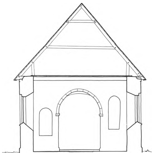
Fig. 7. Tværsnit 1:150 gennem skib, set mod øst. Målt af Henrik Gram og Søren Gottfred Petersen 1978; enkelte rettelser ved NJP 1986. Tegnet af MN 1987. — Querschnitt durch das Schiff nach Osten.
