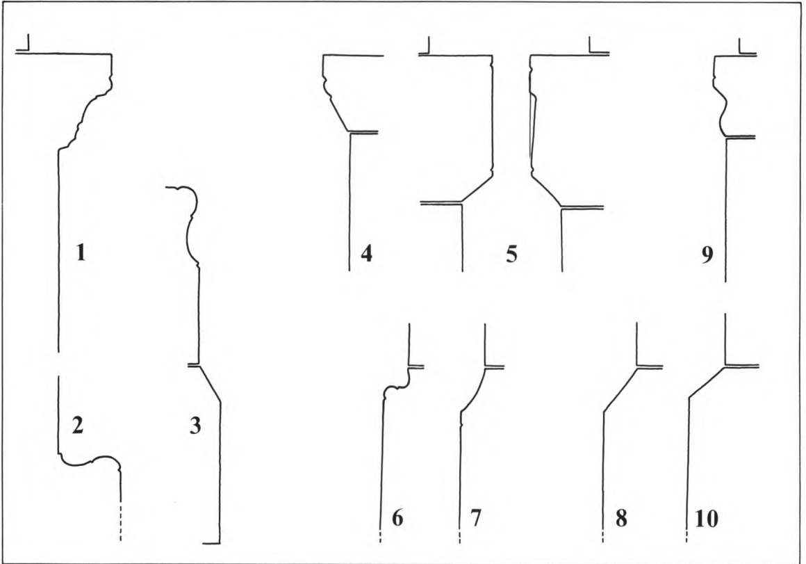
ROMANSKE BYGNINGSPROFILER i Vester Horne herred, 1:10, målt af EIM og NJP, tegnet af MN 1985. Fig. 1-3: Janderup. 1. Korbuekrægbånd. 2. Korbuesokkel. 3. Bygningsokkel. 4-5: Ål. 4. Alterbordsgesims. 5. Korbuekrægbånd. 6-7: Ovtrup, bygningsokkel. 6. Korets og skibets østende. 7. Skibets vestende. 8-10: Billum. 8. Bygningsokkel i apsis og kor. 9. Korbuekrægbånd. 10. Korbuesokkel. Alt i granit, fig. 9. dog i tuff. — Romanische Gebäudeprofile in der Harde von Vester Horne, 1:10, vermessen von EIM und NJP, gezeichnet 1985 von MN. Fig. 1-3: Janderup. 1. Triumphbogenkranzgesims. 2. Triumphbogensokkel. 3. Gebäudesokkel. 4-5: Ål. 4. Altargesims. 5. Triumphbogenkranzgesims. 6-7: Ovtrup, Gebäudesokkel. 6. Ostende des Chors und Schiffs. 7. Westende des Schiffs. 8-10: Billum. 8. Gebäudesokkel in Apsis und Chor. 9. Triumphbogenkranzgesims. 10. Triumphbogensokkel. Alles in Granit, fig. 9. jedoch in Tuff.
