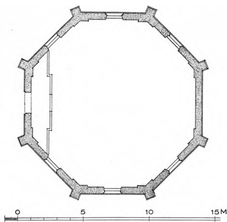
Fig. 2. Nyord. Plan. 1: 300. Maalt af C. A. Jensen 1930 (C. G. Schultz 1934).
