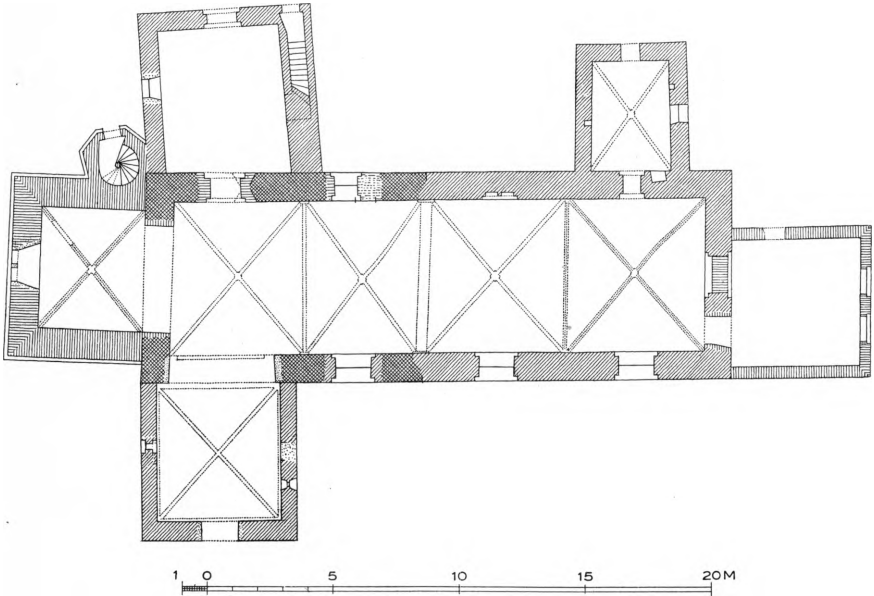
Fig. 2. Magleby. Plan. 1:300. Maalt af Helge Holm 1915 (C. G. Schultz 1932).
