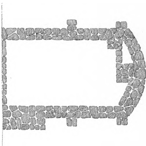
Fig. 5. Vordingborg. Helligaandshus. Plan, 1:300, maalt af J. Kornerup 1884.
