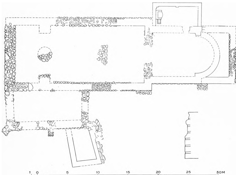
Fig. 3. Vordingborg Slotskirke. Plan, 1:300, af Fundamenter. Efter Opmaalinger af J. B. Løffler og Otto Smith (Aage Roussell). Sokkelprofilen er gengivet i 1:10.
