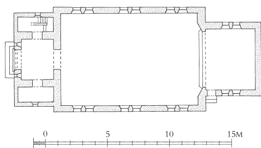
Fig. 3. Plan. 1:300. Målt af Ebbe Lehn Petersen 1988, suppleret af Anders C. Christensen og tegnet af Freerk Oldenburger 2023. Signaturforklaring s. 11. – Plan. Key on p. 11.
