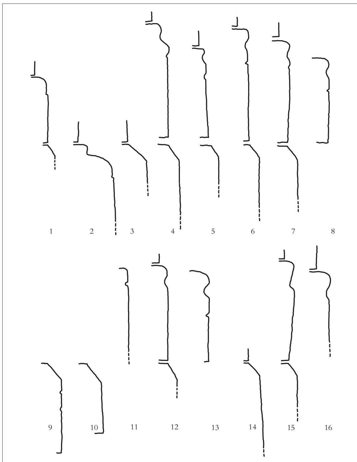
ROMANSKE BYGNINGSSOKLER i Vends Herred, af granit. 1:10. Målt af Kirstin S. Eliassen og tegnet af Mogens Vedsø 2023. 1. Kauslunde. 2-3. Vejlby (kor og skib). 4. Asperup. 5. Brenderup. 6. Fjelsted. 7. Gelsted. 8-11. Rørup (genanvendte). 12. Balslev. 13. Ejby (genanvendt). 14. Gamborg. 15-16. Udby (kor og skib). – Romanesque base profiles in granite.
