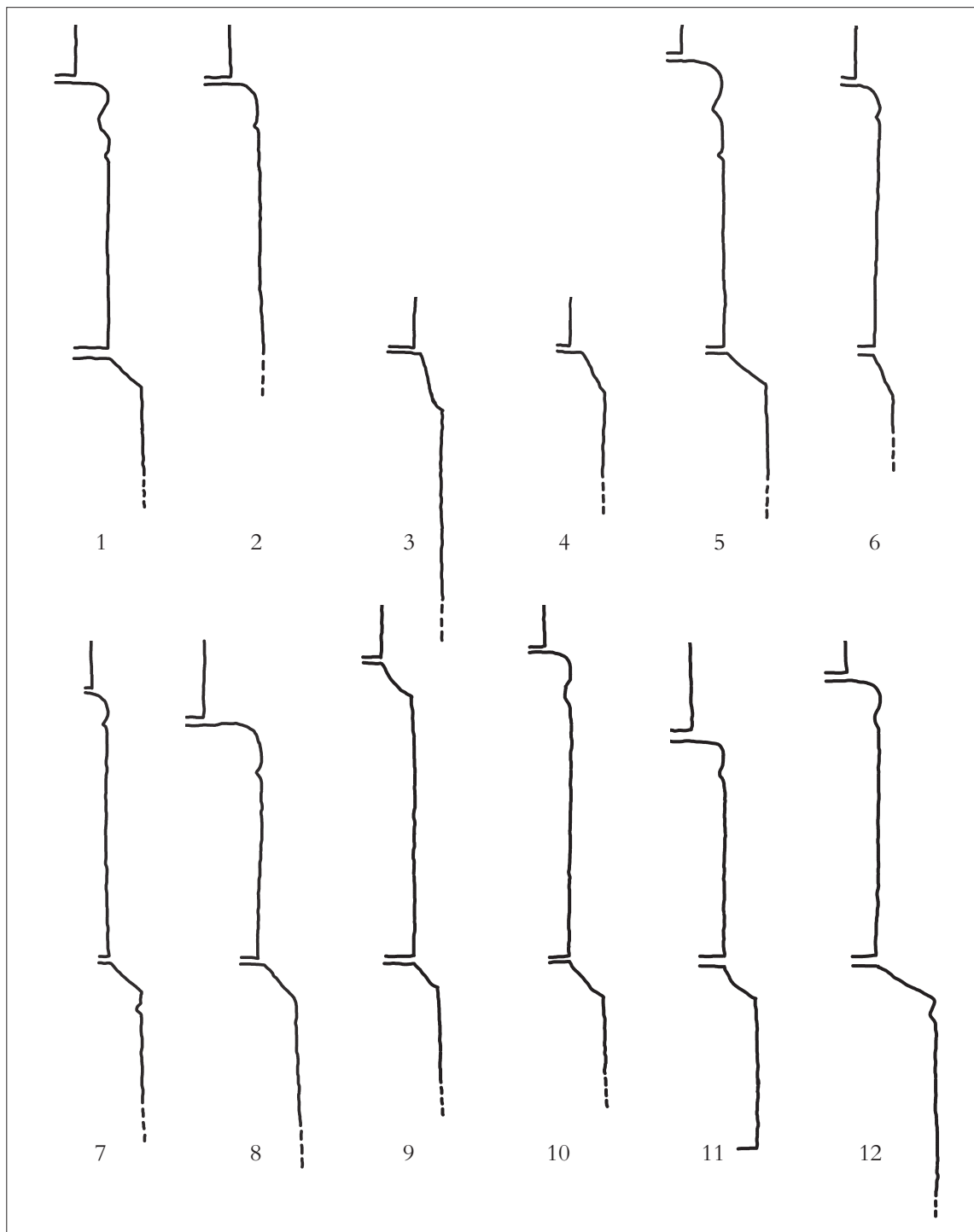
ROMANSKE BYGNINGSSOKLER i Skovby Herred, af granit. 1:10. Målt af Kirstin S. Eliassen og tegnet af Mogens Vedsø 2020. 1. Skovby, apsis, kor og skib. 2. Skovby, fire kvadre i skib øst for våbenhus. 3. Guldbjerg, genanvendte apsiskvadre. 4. Nørre Sandager, skib. 5. Ejlby, apsis, kor og skib. 6. Melby, apsis. 7. Særslev, kor. 8. Hårslev, skib. 9. Veflinge, skib (nordside). 10. Veflinge, skib (sydside, vestre afsnit). 11. Vigerslev, genanvendt i langhuskor. 12. Sønder sø, kor. – Romanesque base profiles in granite.
