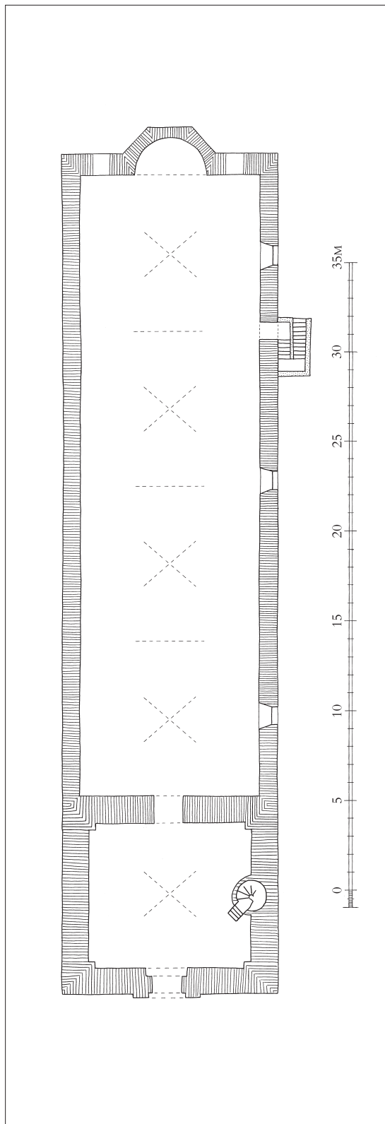
Fig. 4. Rekonstrueret grundplan med antydning af fagdeling og overhvelvning (øst opad). 1:300. Baseret på gengivelse af kirken i en grundtegnning over herregården Kjørup, udført af tømmermester Johan Adam Weinbrenner, Odense, 1781. Tegnet af Freerk Oldenburger 2019. Signaturforklaring s. 11. – Reconstructed ground plan with a hint of bay division and vaulting (eastwards), based on the recording of the church on the plan of the manor house of Kjørup, by master carpenter Johan Adam Weinbrenner, Odense, 1781. Key on p. 11.
