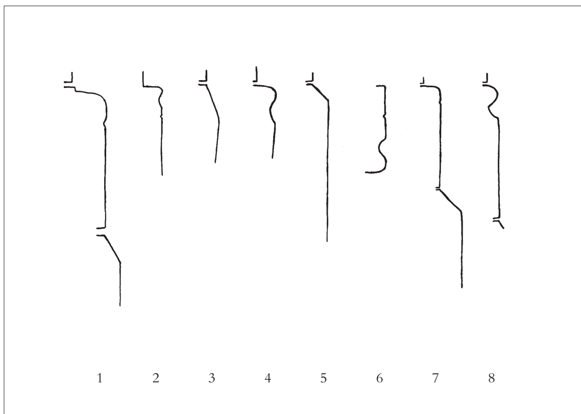
ROMANSKE BYGNINGSSOKLER m.m. i Lunde Herred, af granit. 1:10. Målt og tegnet af Kirstin Eliassen 2018. 1. Norup, kor. 2-3. Otterup, kor. 4. Otterup, skib. 5. Hjadstrup. 6. Hjadstrup, kragbånd (her gengivet omvendt). 7. Lunde, kor. 8. Lunde, skib. – Romanesque base profiles in granite.
