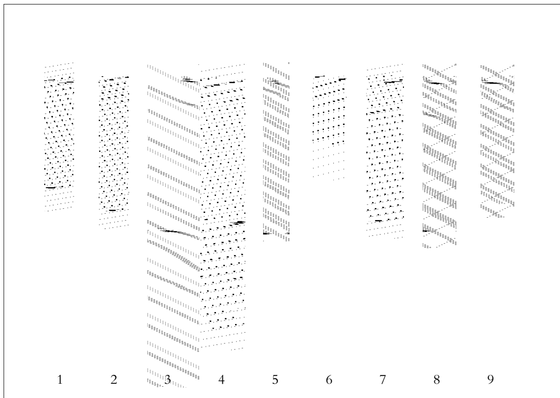
ROMANSKE BYGNINGSSOKLER i Bjerge Herred, af granit. 1:10. Målt og tegnet af Martin Wangsgaard Jürgensen, suppleret af Kirstin Eliassen 2017. 1. Drigstrup. 2. Munkebo. 3. Kølstrup, kor. 4. Kølstrup, skib. 5. Marslev. 6. Revninge. 7. Mesinge. 8. Dalby, kor. 9. Dalby, skib. – Romanesque base profiles in granite.
