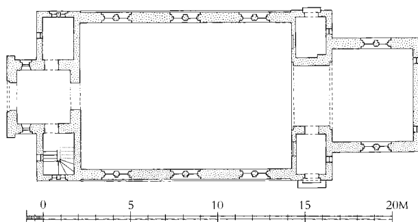
Fig. 4. Plan. 1:300. Målt af J. Vilh. Petersen 1906, suppleret af Kirstin Eliassen og tegnet af Merete Rude 2015. – Ground plan.
