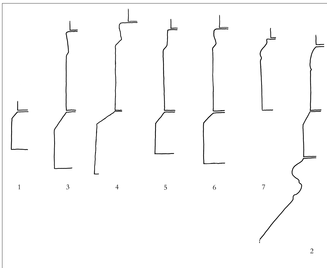
ROMANSKE BYGNINGSSOKLER i Odense Herred, af granit, 1:10. Målt og tegnet af Martin Wangsgaard Jürgensen 2013. 1. Pårup. 2. Sanderum. 3. Stenløse. 4. Verninge. 5. Tommerup. 6. Brylle. 7. Vissenbjerg. – Romanesque base profiles in granite.
