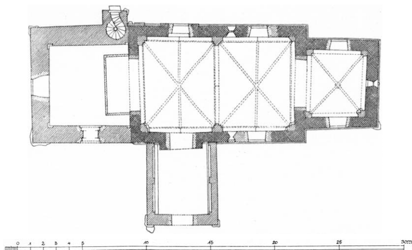
Fig. 2. Stadager. Plan. 1:300. Målt af Tove Bojesen 1952.
